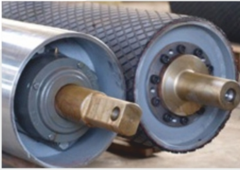
Pulley Lagging
