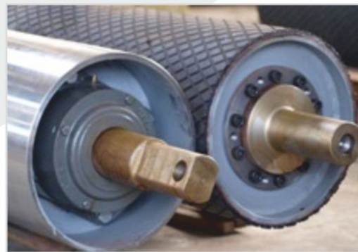
Pulley Laggings
